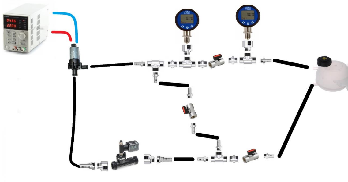
Pav. 1. Hidraulini siurblio parametų demonstravimo schema
